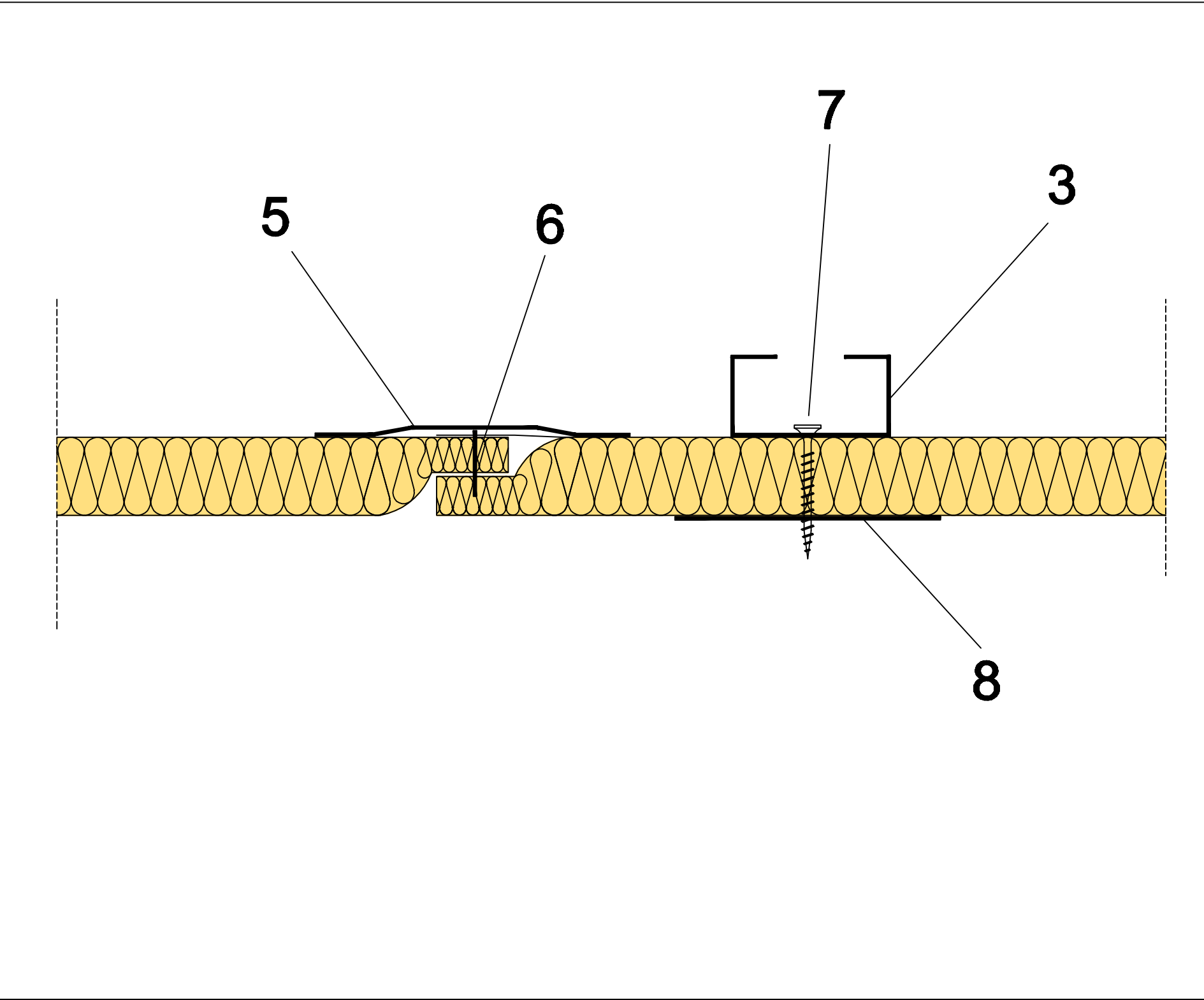
DETALLE UNIÓN DE SECCIONES DE CONDUCTO AUTOPORTANTE
