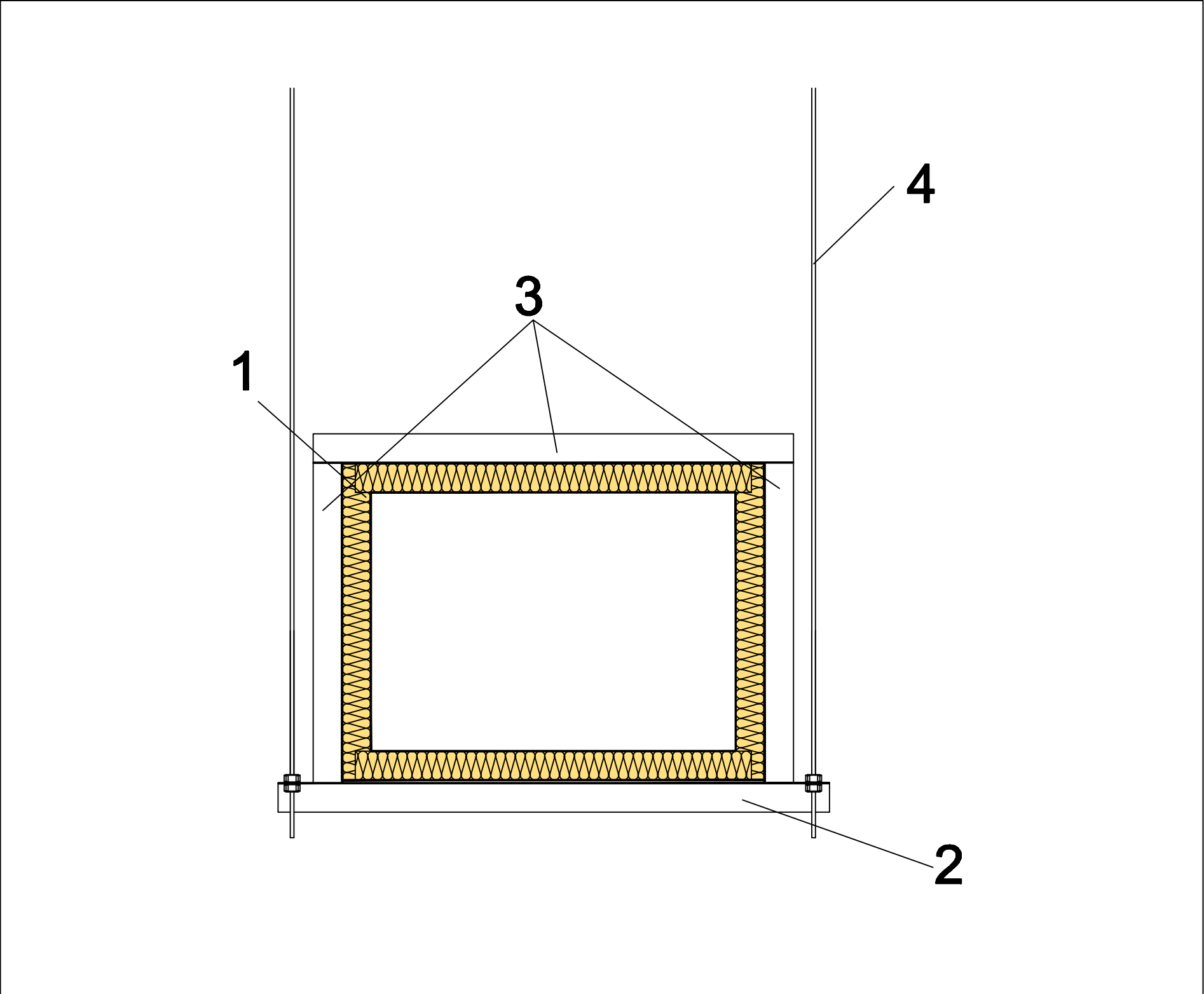
SECCIÓN TRANSVERSAL
