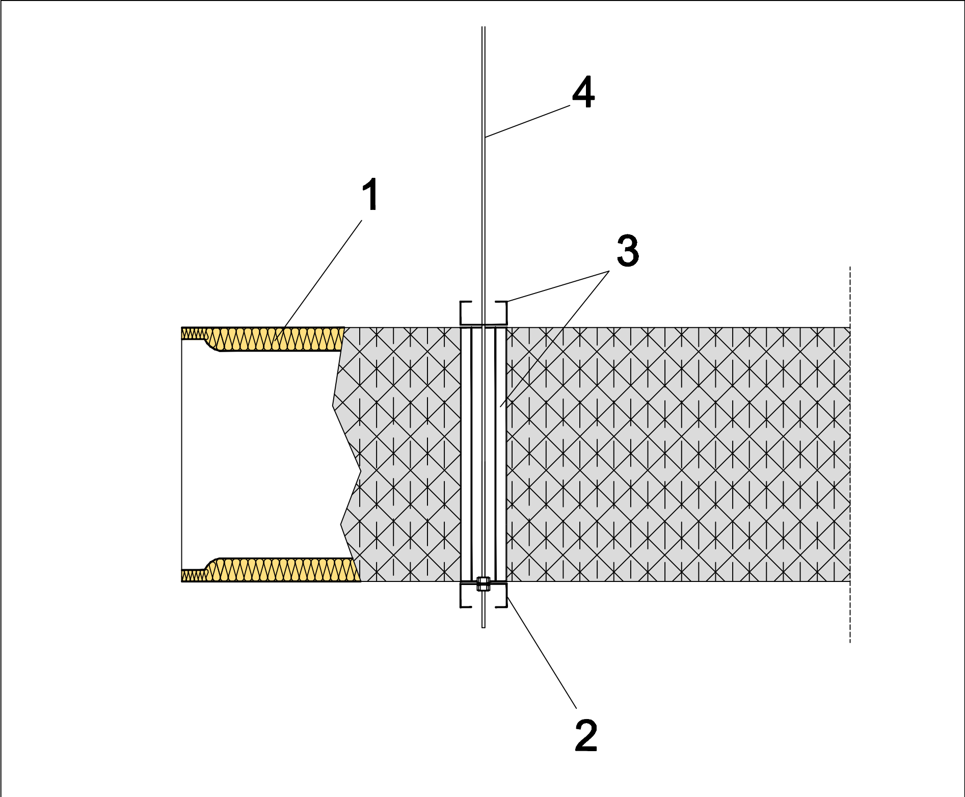
SECCIÓN LONGITUDINAL
