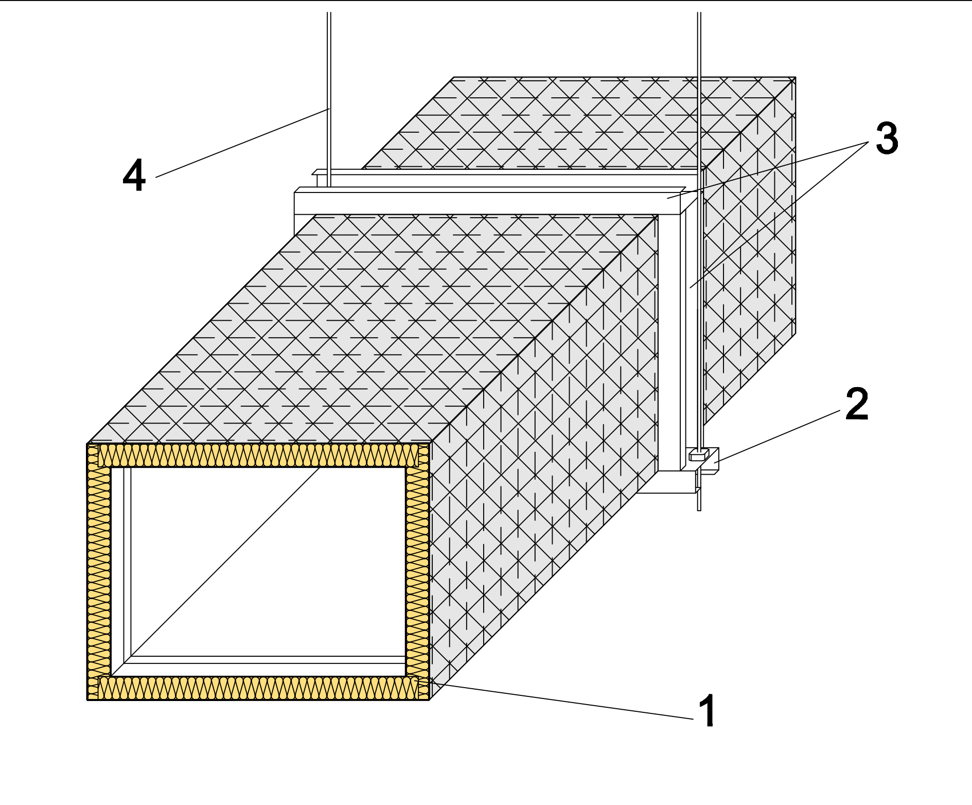
CONDUCTO AUTOPORTANTE CON REFUERZOS
