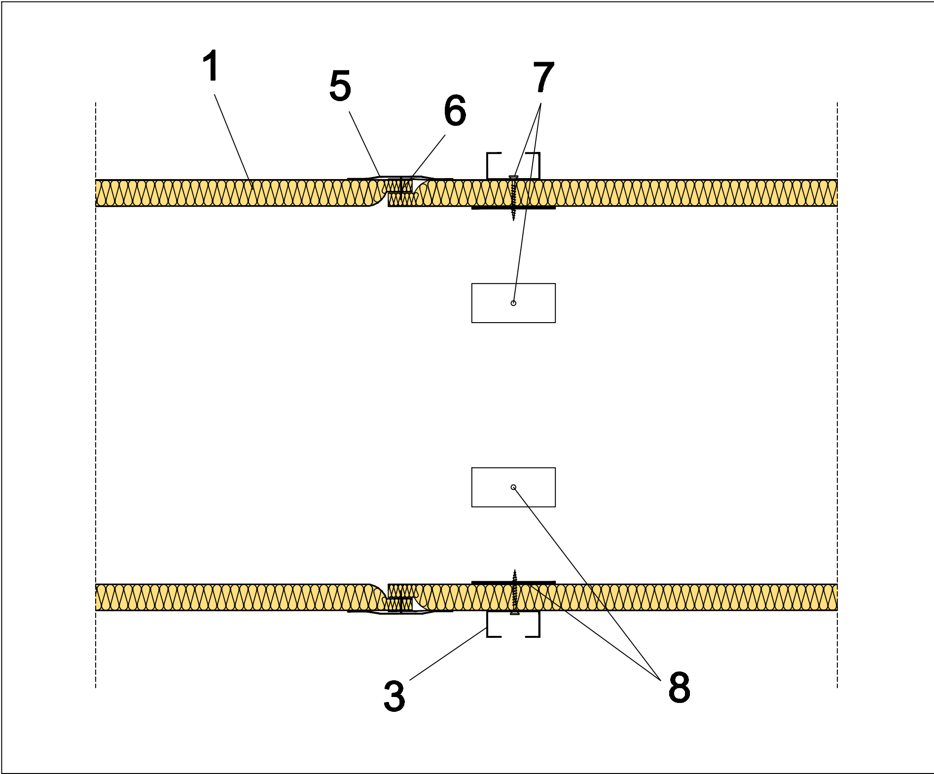
REFUERZOS INTERIORES EN CONDUCTOS. SECCIÓN LONGITUDINAL.
