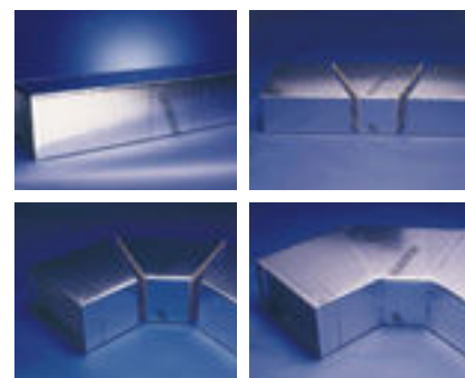
CLIMAVER: ventajas del sistema completo:
