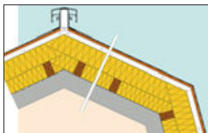
Estructura de tejado con diferentes pendientes
