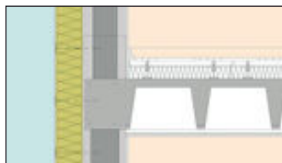
Sistema de aislamiento térmico con paneles de lana mineral ISOVER
