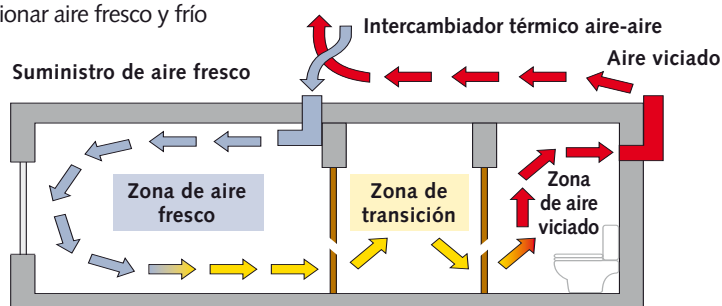
Sistema de ventilación simplificado
