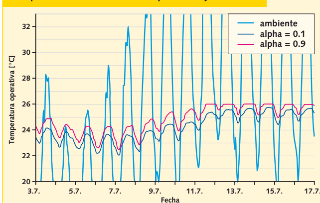
Temperatura sala de estar en planta baja (Sevilla)
