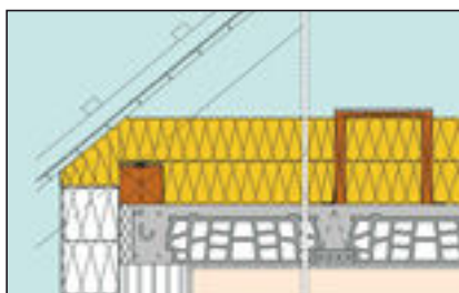
Aislamiento en el techo de la planta superior
