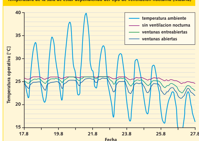
Temperatura de la sala de estar dependiendo del tipo de ventilación nocturna (Madrid)
