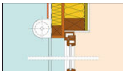
Marcos de madera con elementos para proporcionar sombra en las ventanas
