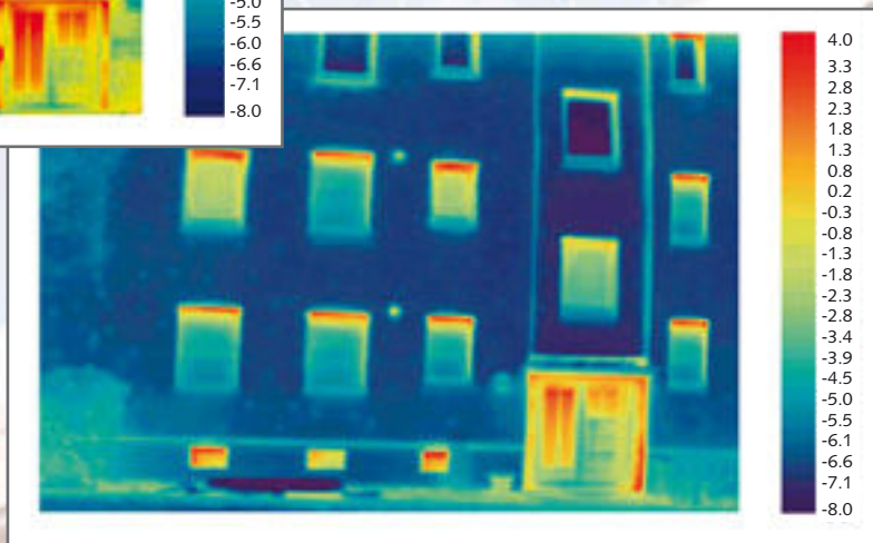
Imagen termográfica – después de la rehabilitación: La pared externa está aislada térmicamente, pero el calor todavía se escapa a través de ventanas y puertas y, sobre todo, por las cajas de persiana.
