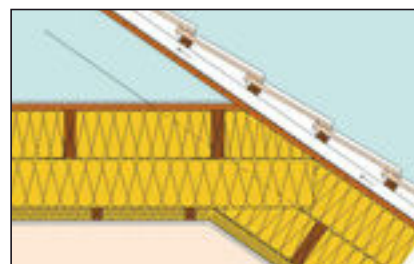
Aislamiento de estructura de madera
