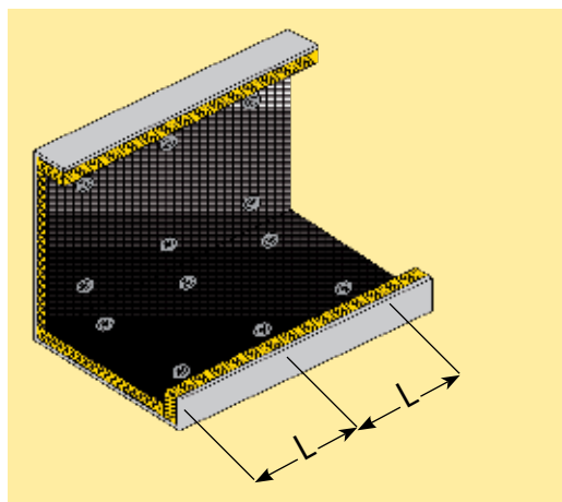
Detalle de colocación de los pernos de fijación.
