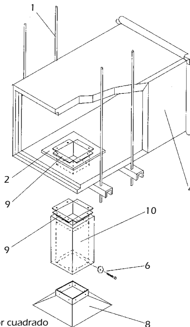
Difusor cuadrado
