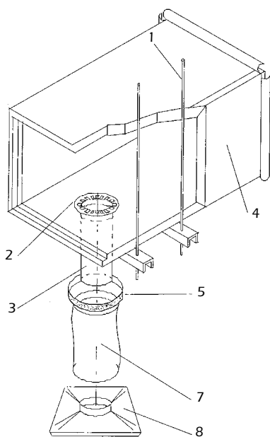
Difusor redondo
