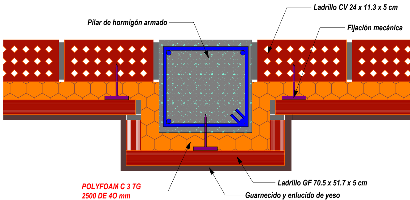
FACHADA DOBLE HOJA CON POLYFOAM C 3 TG 2500
