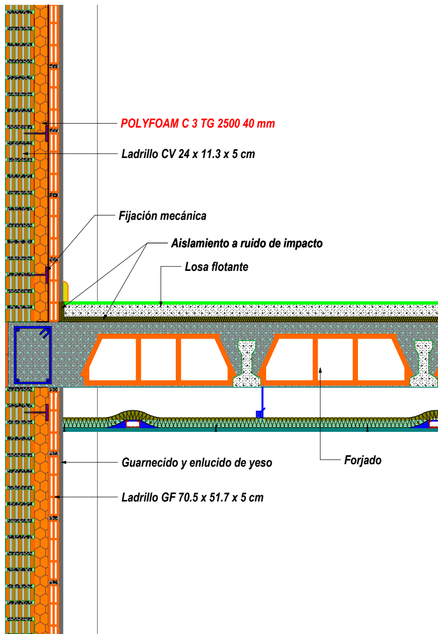
FACHADA DOBLE HOJA CON POLYFOAM C 3 TG 2500
