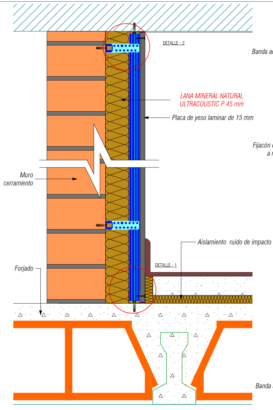
TRASDOSADO AUTOPORTANTE CON ULTRACOUSTIC P
