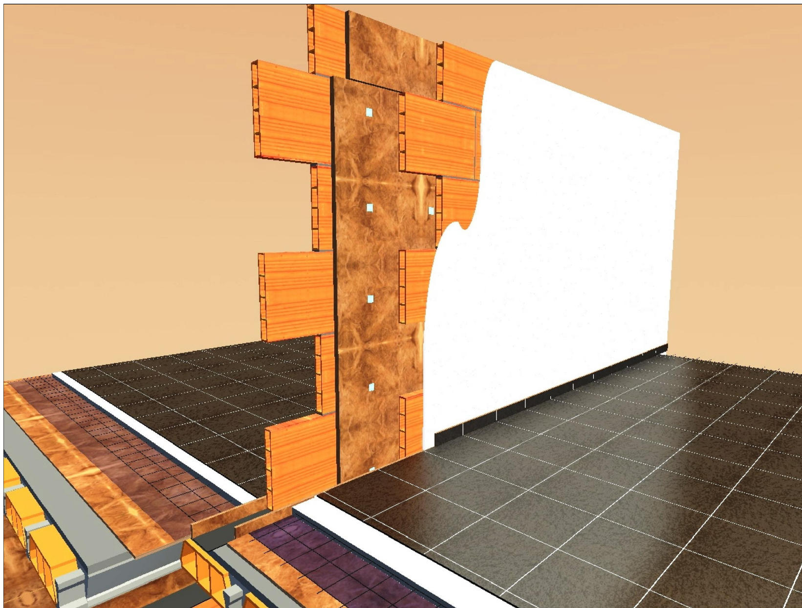
PARED DE LADRILLO CON DOBLE HOJA LGF 70 mm Y ULTRACOUSTIC G 45 mm
