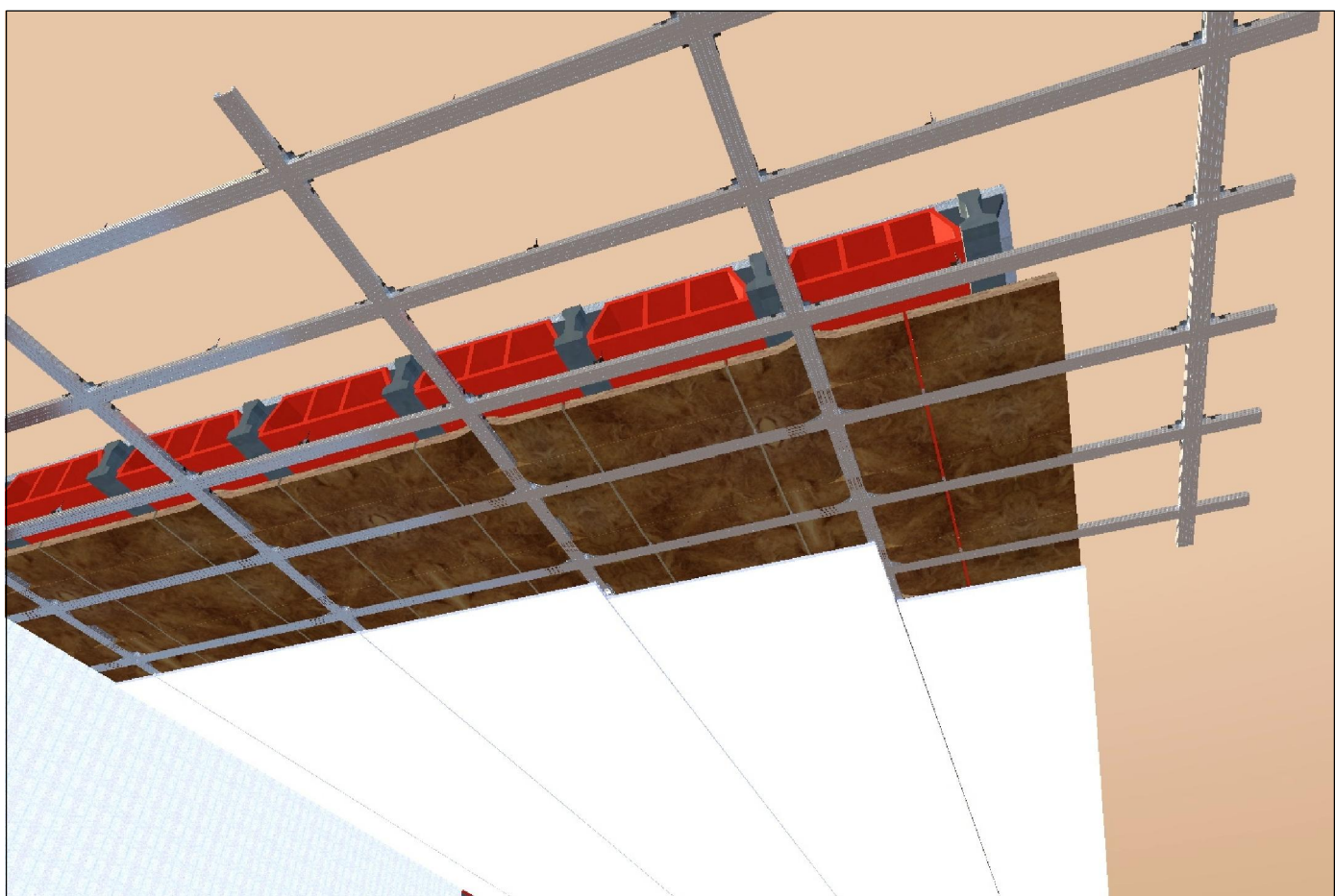
FALSO TECHO CIEGO CON ULTRACOUSTIC R
