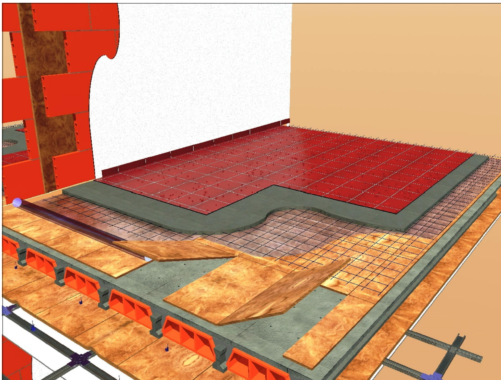
SUELO FLOTANTE CON ULTRACOUSTIC SUELOS TPT 01
