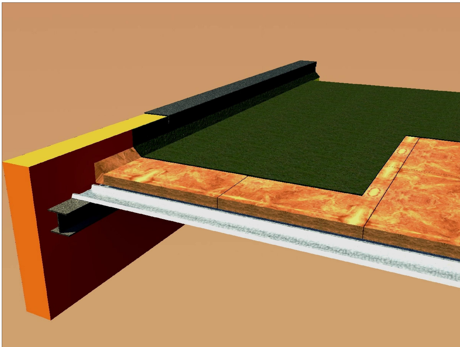
CUBIERTA DECK CON PANEL CUBIERTA PLUS
