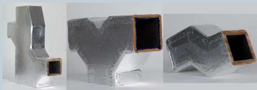
Piezas especiales de una red de conductos realizadas con paneles CLIMACOUSTIC
