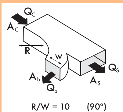
Conducto principal
