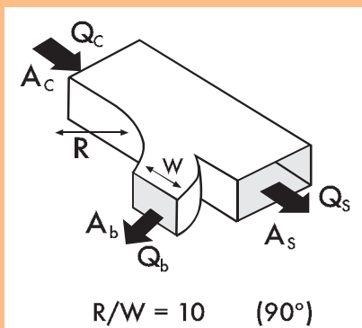
Derivación
