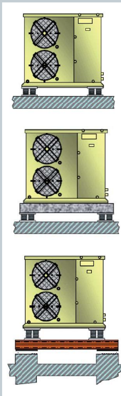
Los sistemas antivibratorios reducen las transmisiones acústicas de las máquinas de acondicionamiento de aire a los elementos constructivos del edificio
