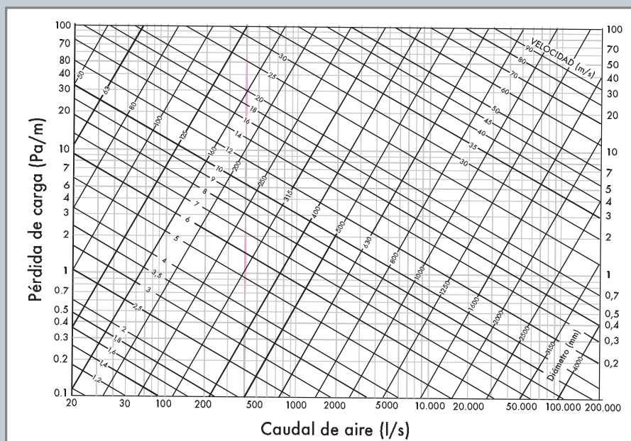
Gráfico de rozamiento de ASHRAE
