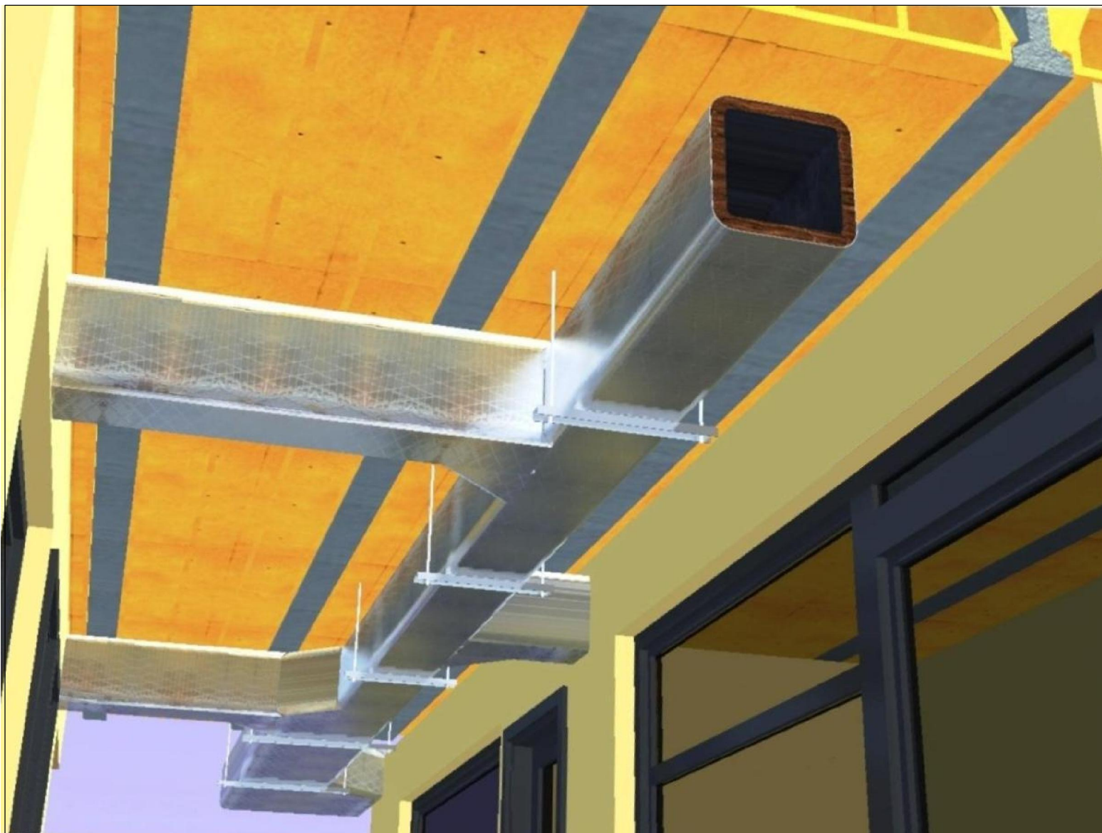
CONDUCTO AUTOPORTANTE RECTANGULAR - CLIMACOUSTIC PANEL AUTOPORTANTE DE LANA MINERAL
