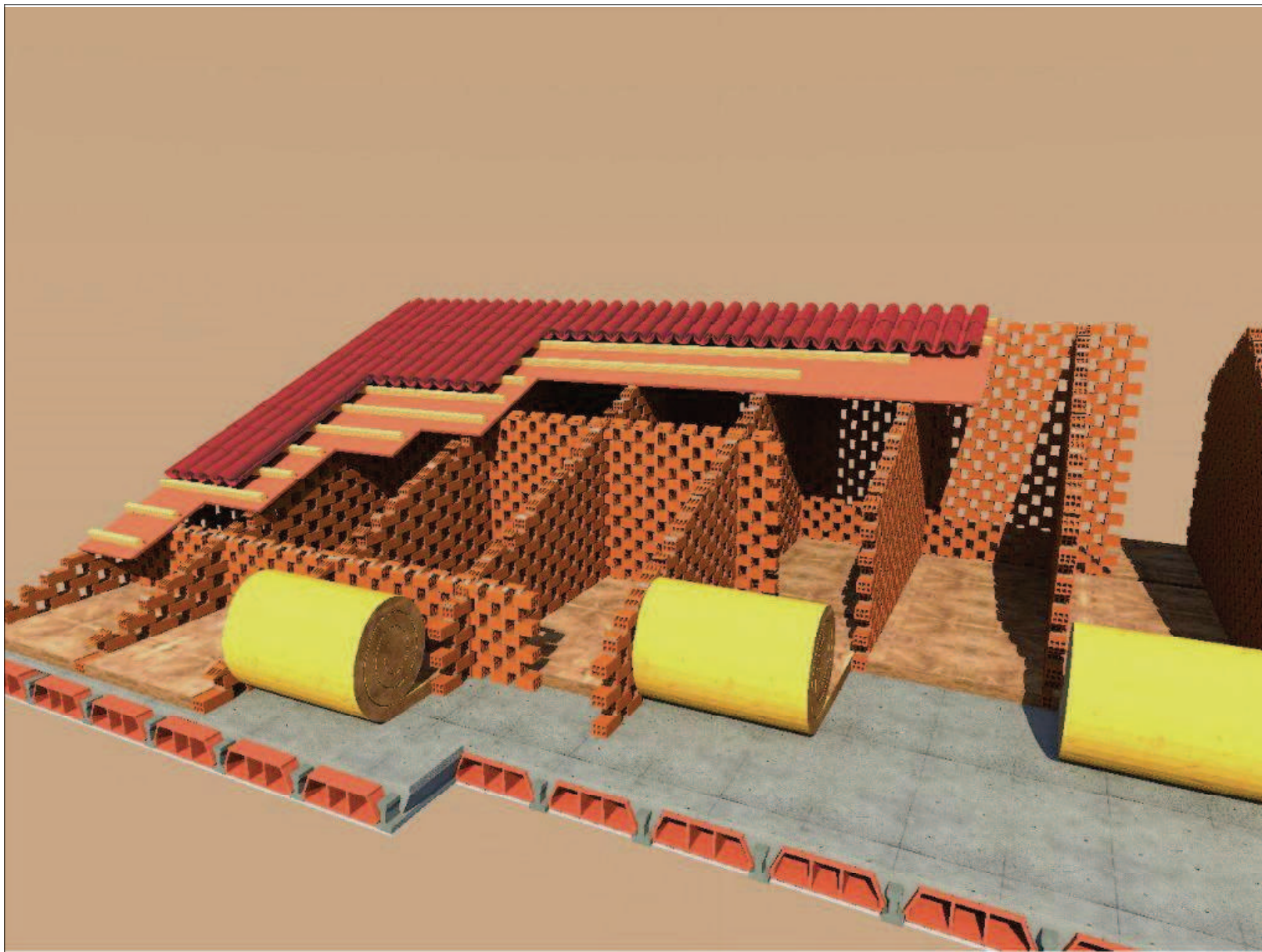
CUBIERTA INCLINADA SOBRE TABIQUILLOS CON MANTA KRAFT (TI 212)
