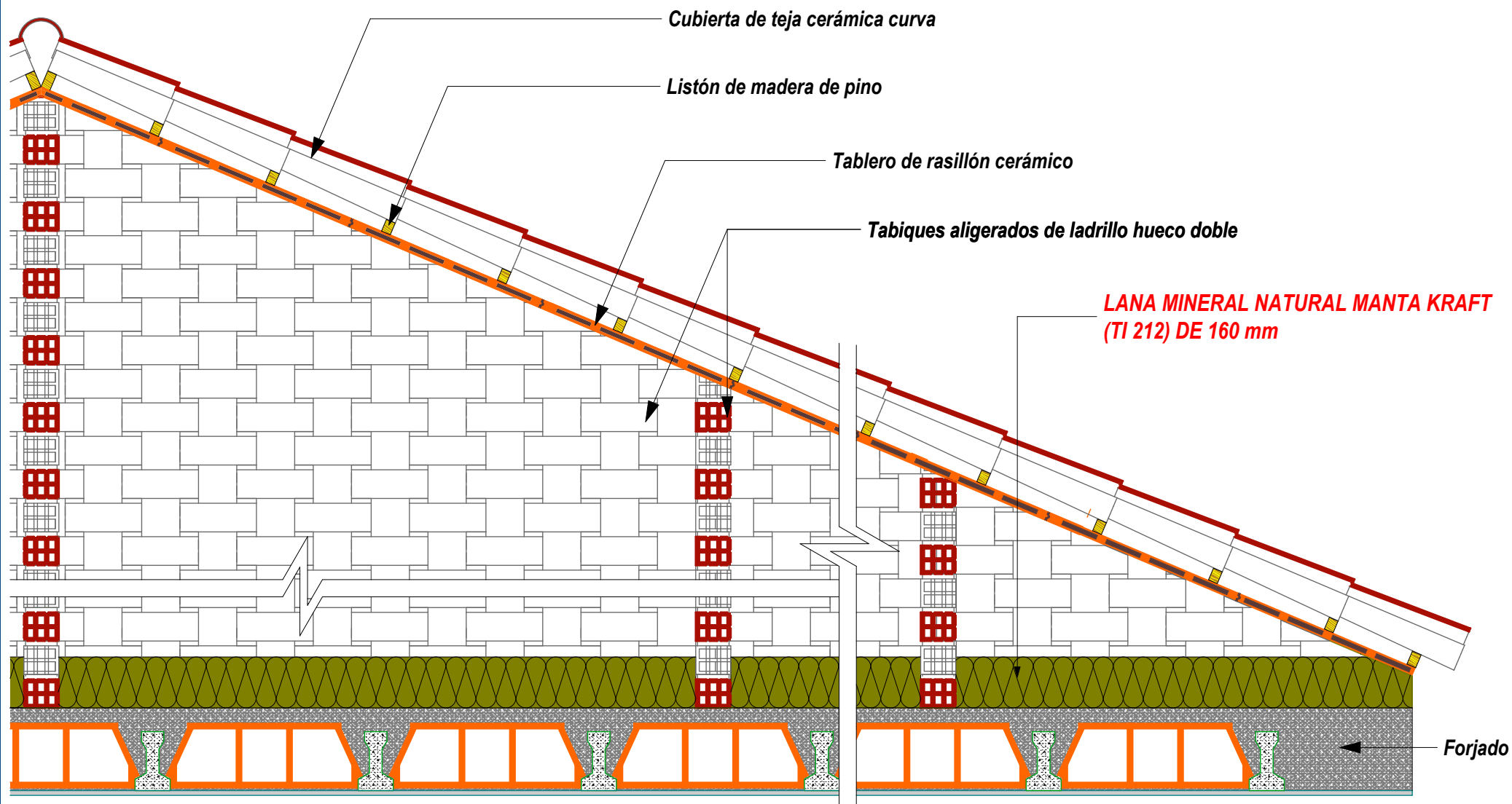
CUBIERTA INCLINADA SOBRE TABIQUILLOS CON MANTA KRAFT (TI 212)
