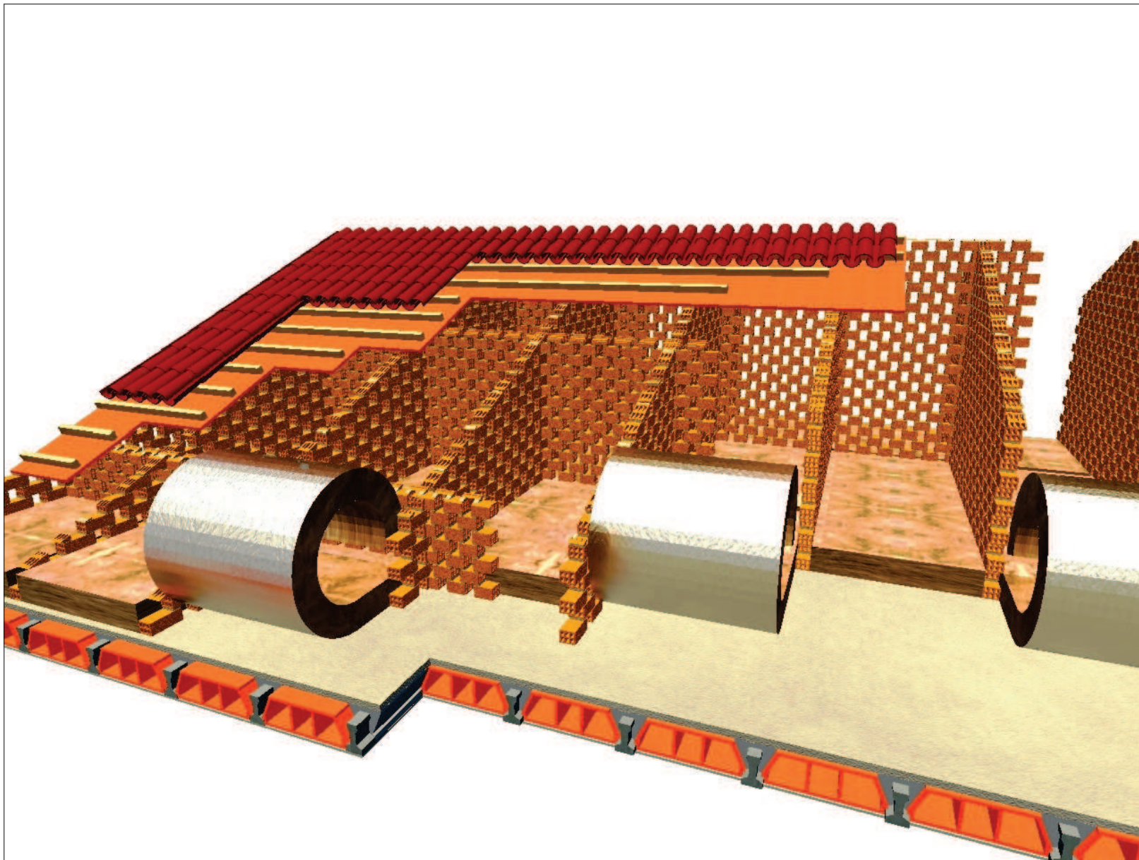
CUBIERTA INCLINADA SOBRE TABIQUILLOS CON MANTA ALUMINIO (TI 312)
