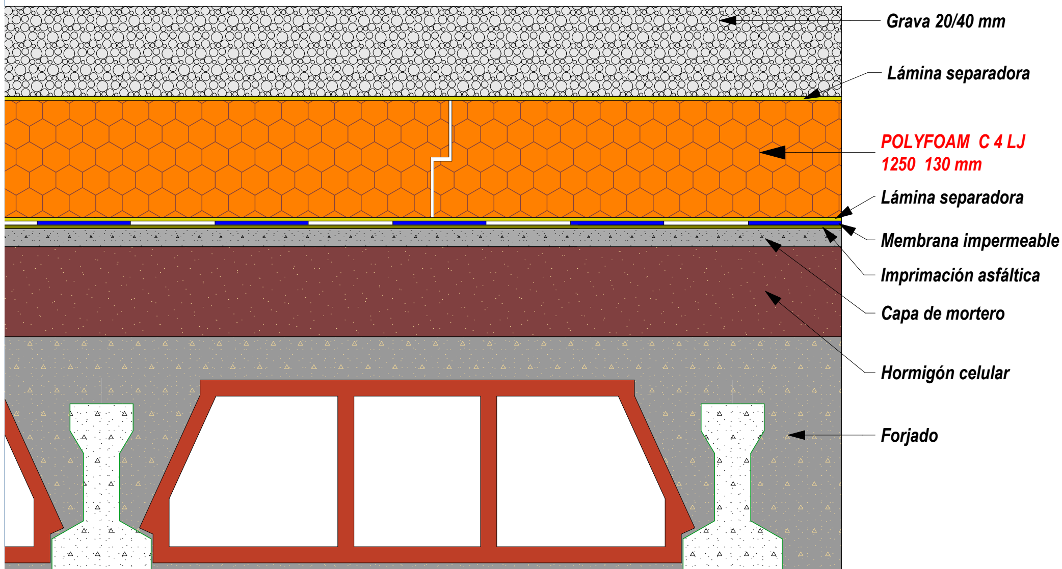
CUBIERTA INVERTIDA CON GRAVA Y POLYFOAM C4 LJ 1250 (no transitable)
