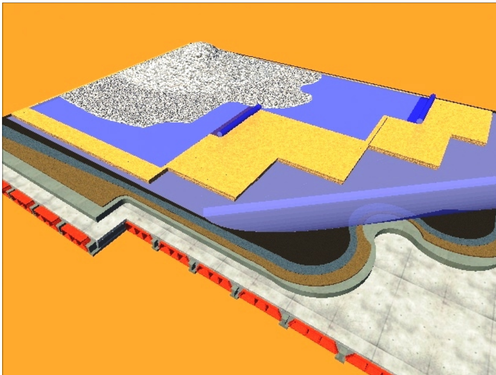
CUBIERTA INVERTIDA CON GRAVA Y POLYFOAM C 4 LJ 1250 (no transitable)
