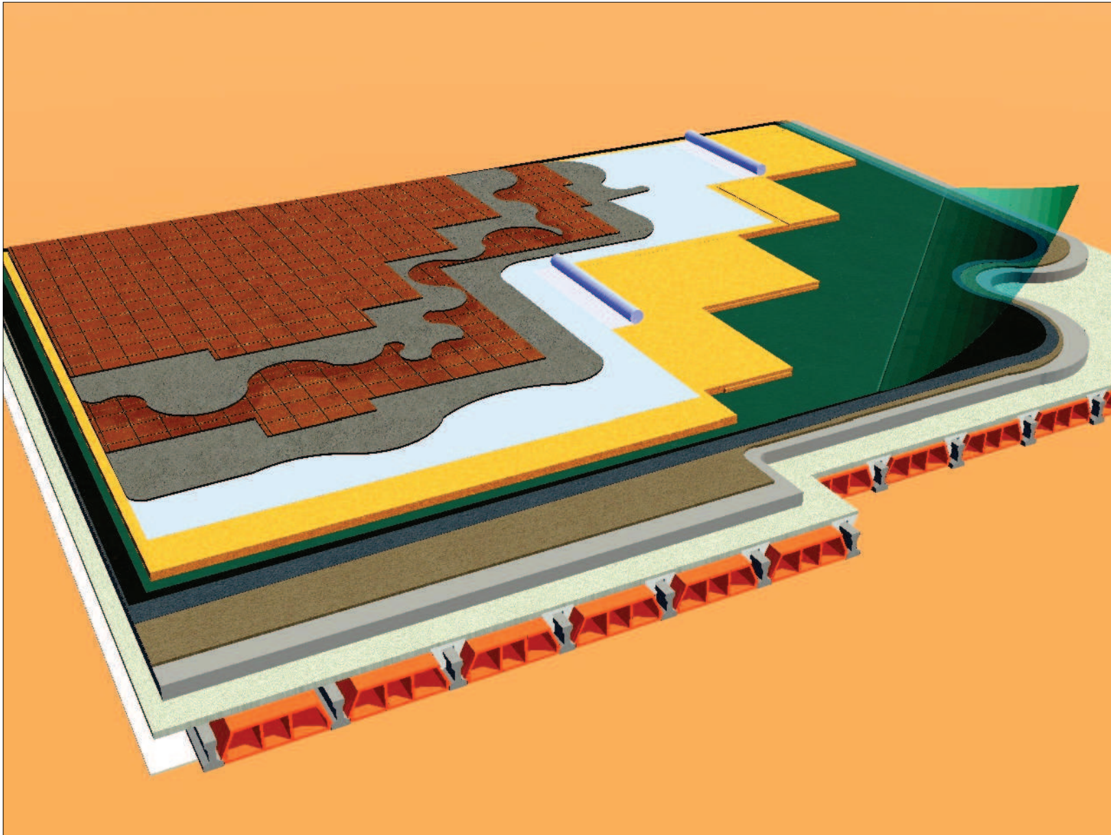
CUBIERTA INVERTIDA CON SOLADO Y POLYFOAM C4 LJ 1250 (Transitable)
