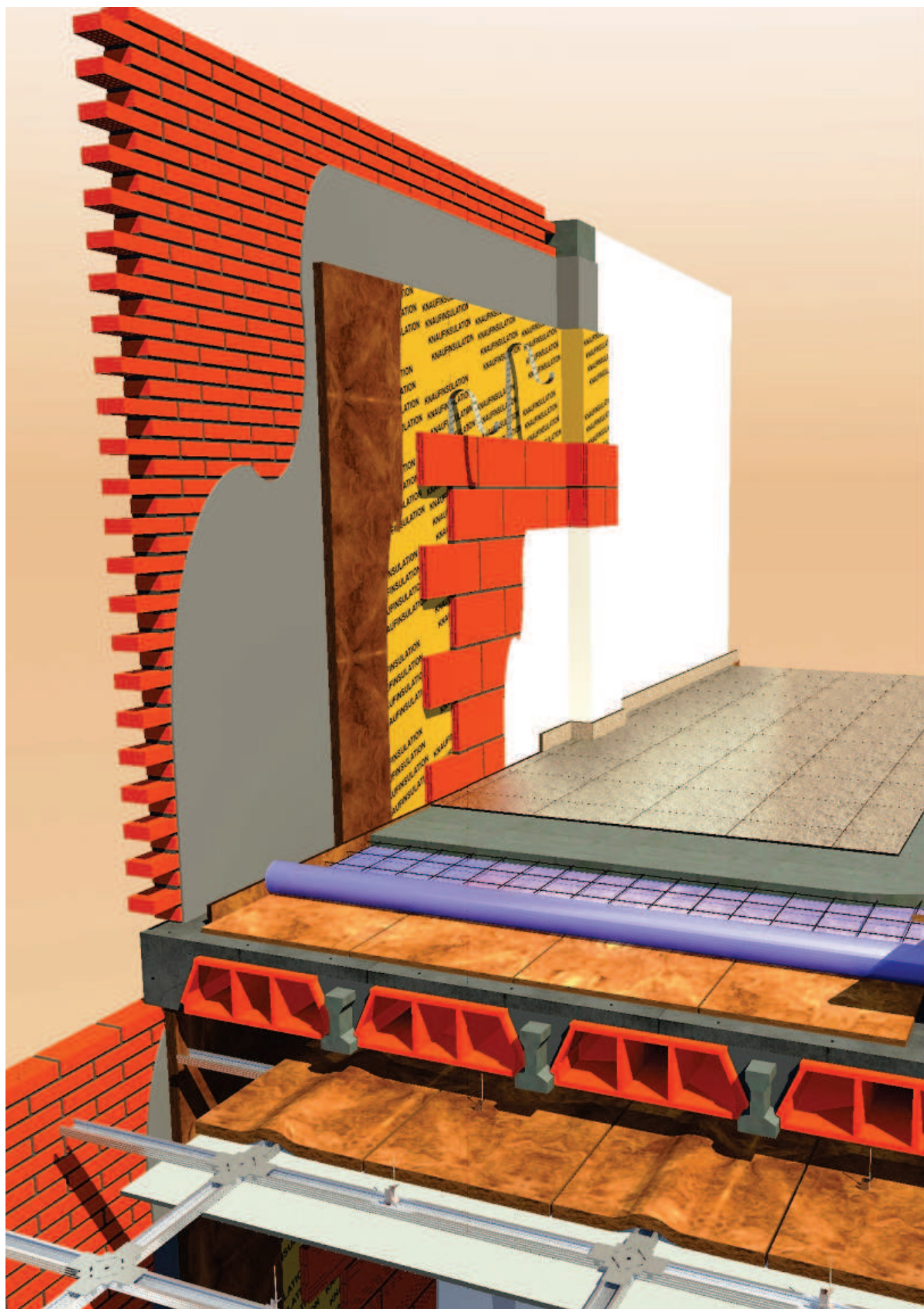
FACHADA DOBLE HOJA CON PANEL PLUS KRAFT EN SISTEMA GECOL-KNAUF INSULATION
