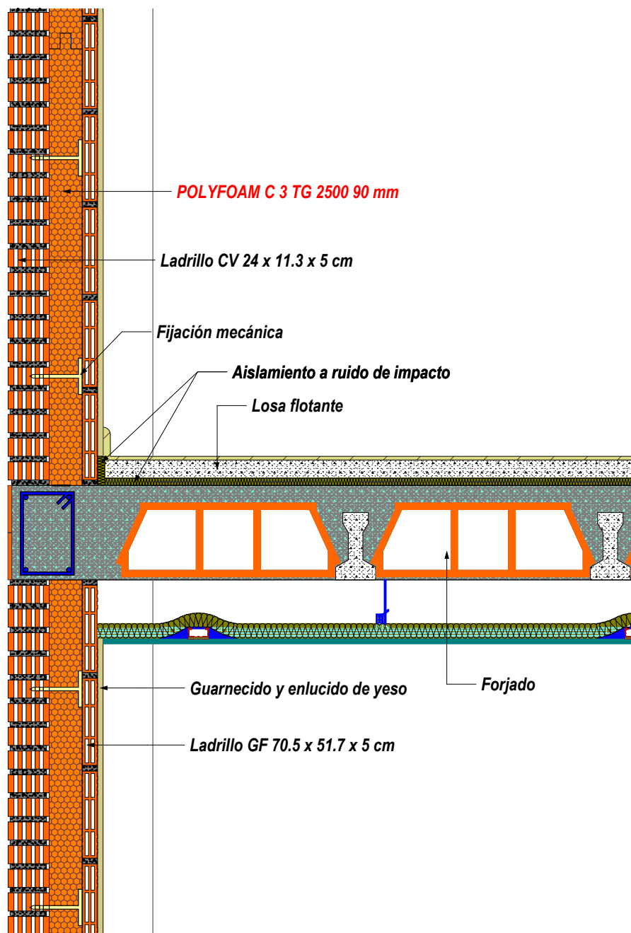
FACHADA DOBLE HOJA CON POLYFOAM C 3 TG 2500
