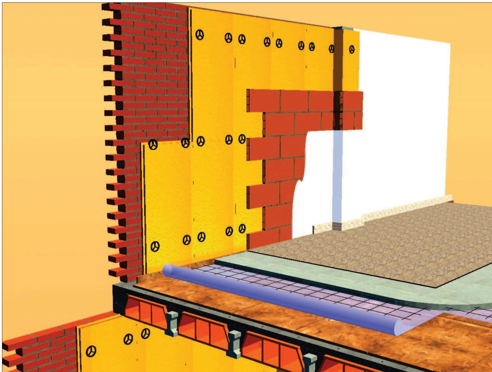
FACHADA DOBLE HOJA CON POLYFOAM C 3 TG 2500
