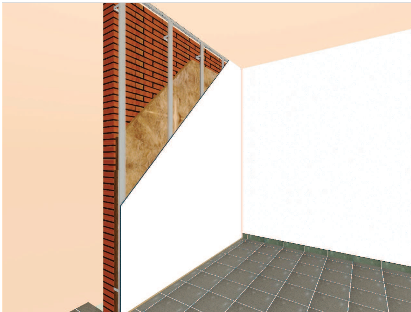
TRASDOSADO AUTOPORTANTE CON ULTRACOUSTIC R
