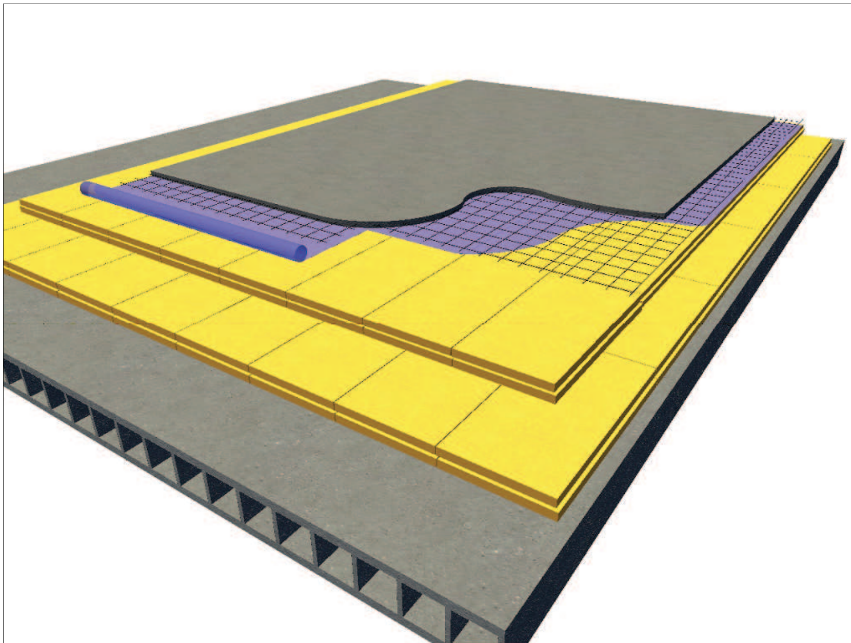
CAMARA FRIGOINDUSTRIAL DE CONGELACION A TEMPERATURA NEGATIVA CON POLYFOAM C 5 LJ 1250
