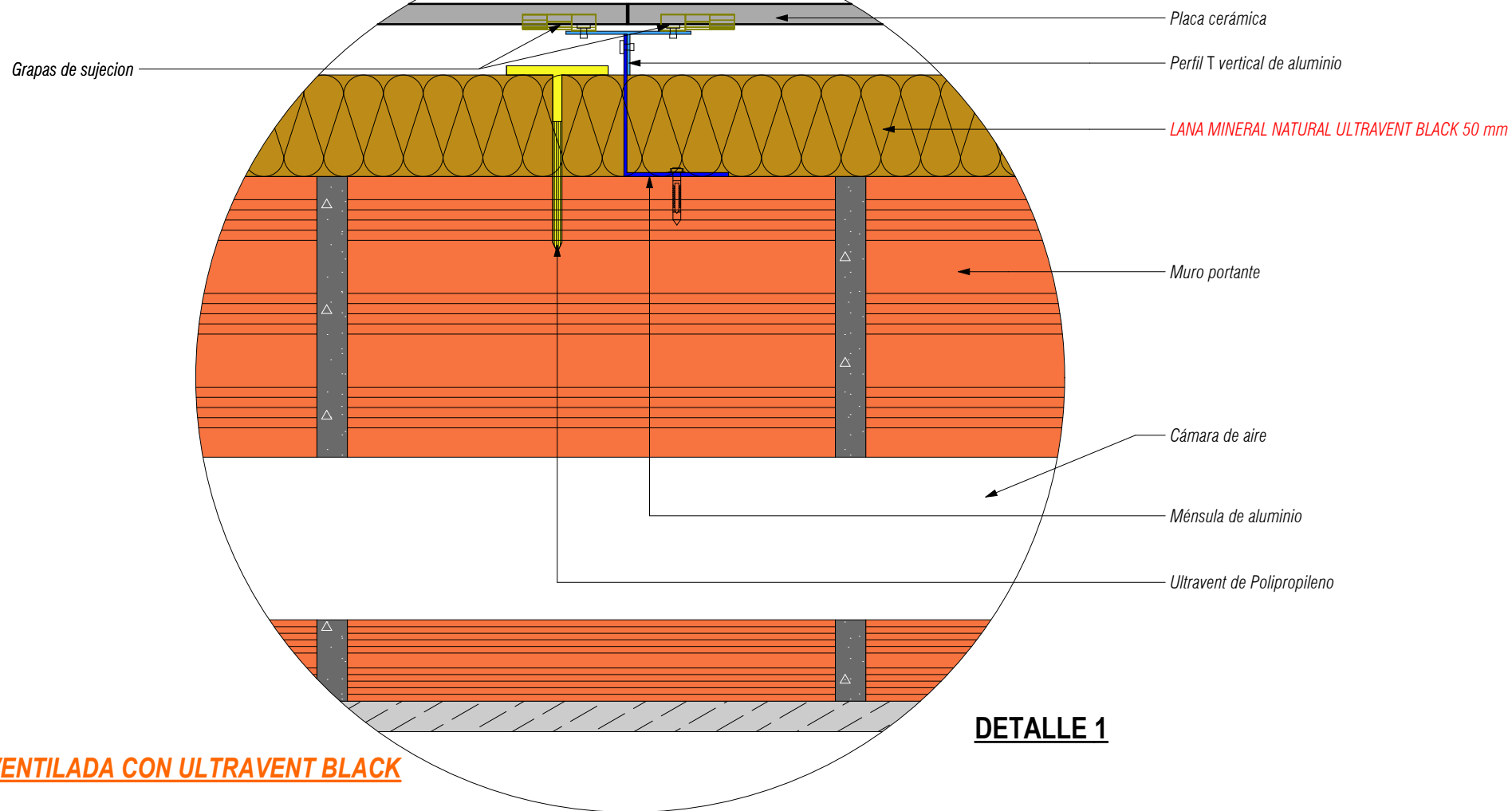
DETALLE 1
