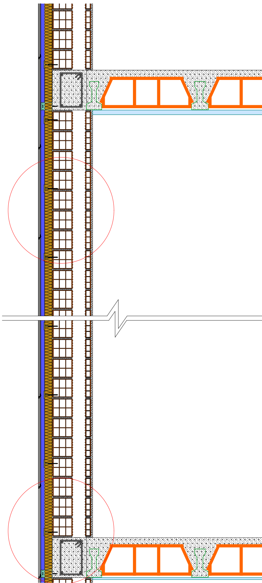
FACHADA VENTILADA CON ULTRAVENT BLACK
