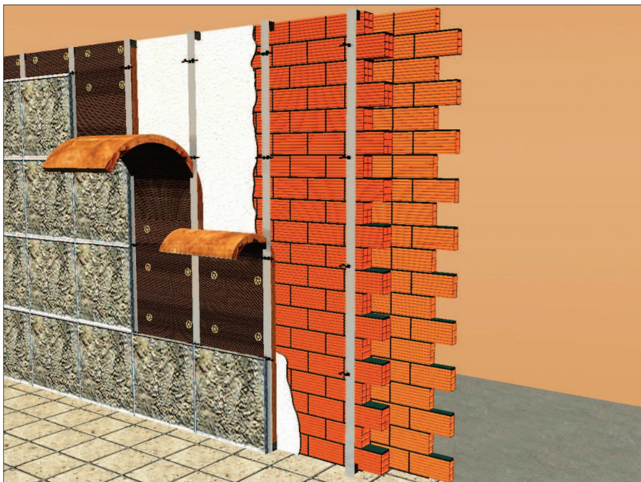
FACHADA VENTILADA CON ULTRAVENT BLACK
