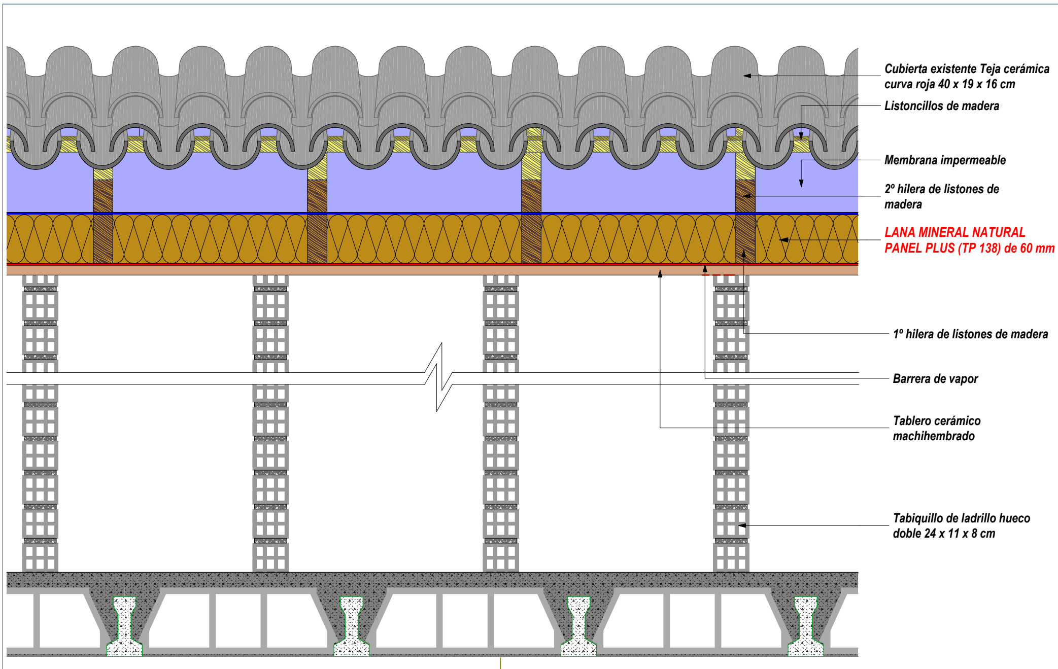
AISLAMIENTO EXTERIOR DE CUBIERTA INCLINADA CON LANA MINERAL NATURAL PANEL PLUS (TP 138)
