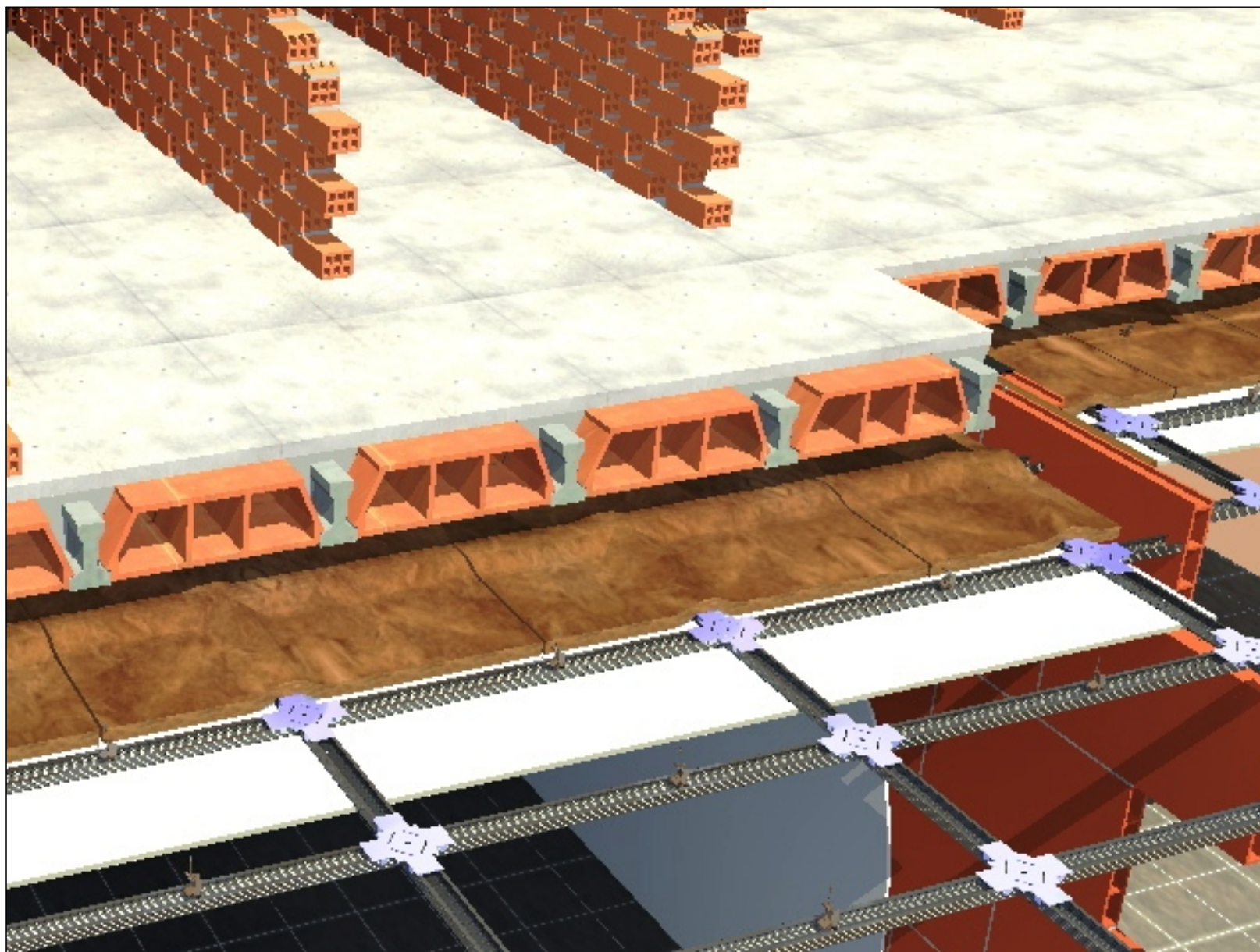
AISLAMIENTO INTERIOR BAJO ULTIMO FORJADO CON LANA MINERAL NATURAL PANEL PLUS (TP 138)
