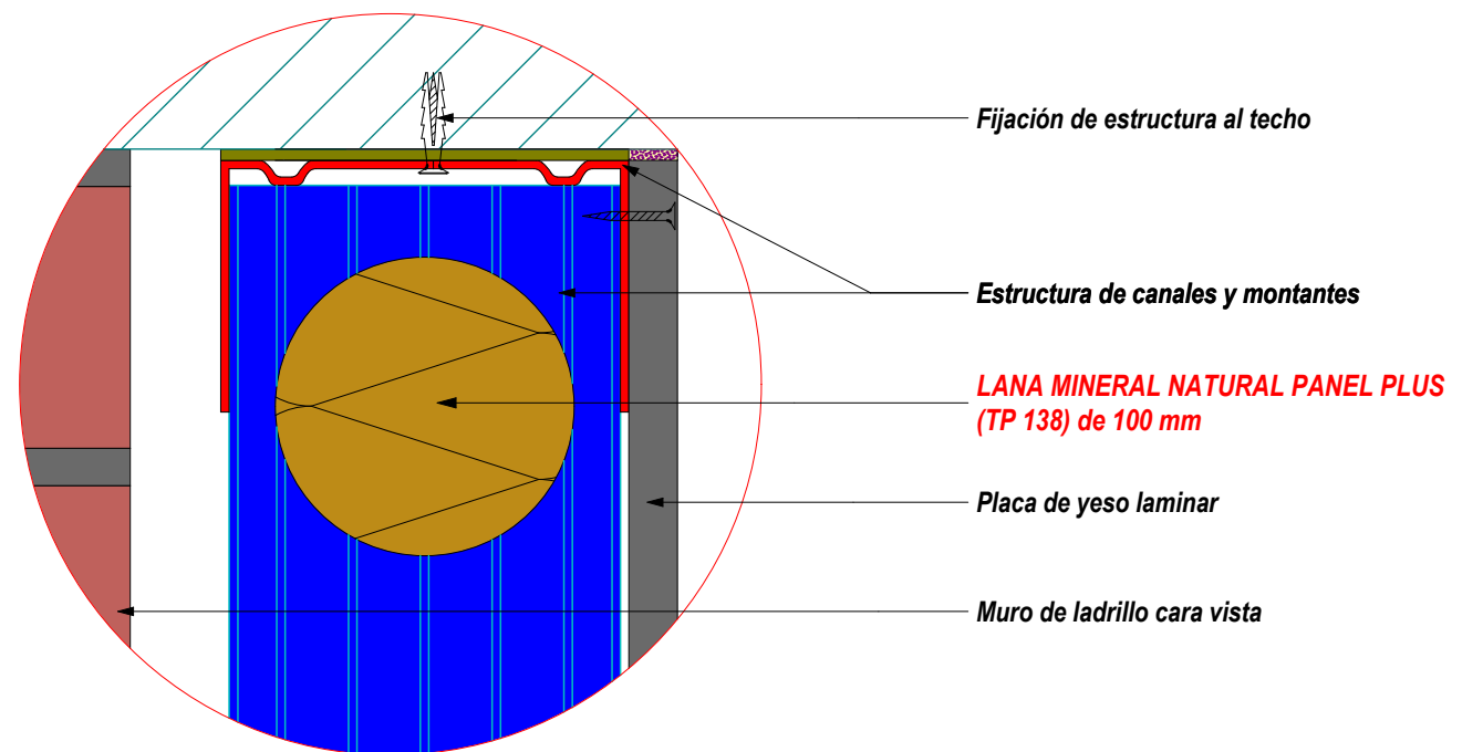
DETALLE - 3
