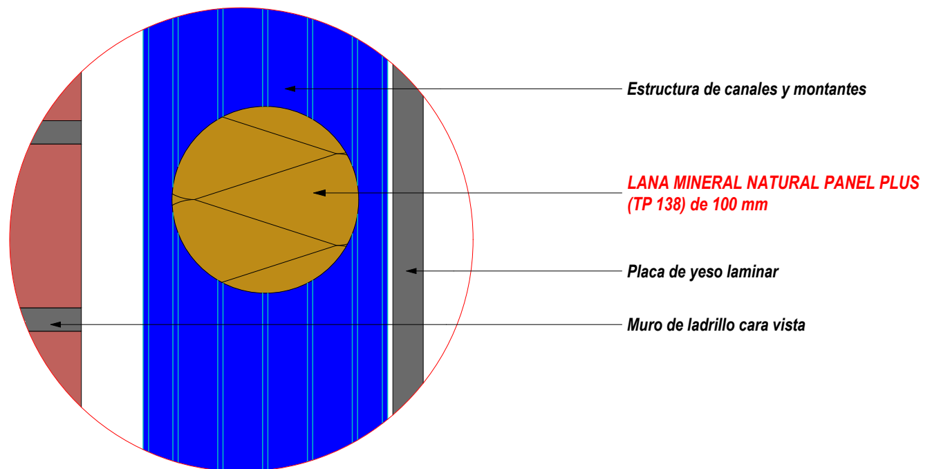
DETALLE - 2
