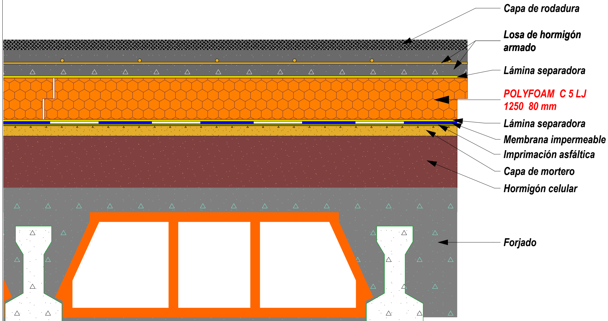
CUBIERTA INVERTIDA PARKING CON POLYFOAM C 5 LJ 1250
