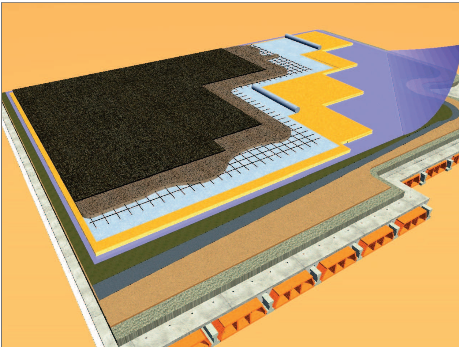
CUBIERTA INVERTIDA PARKING CON POLYFOAM C 5 LJ 1250
