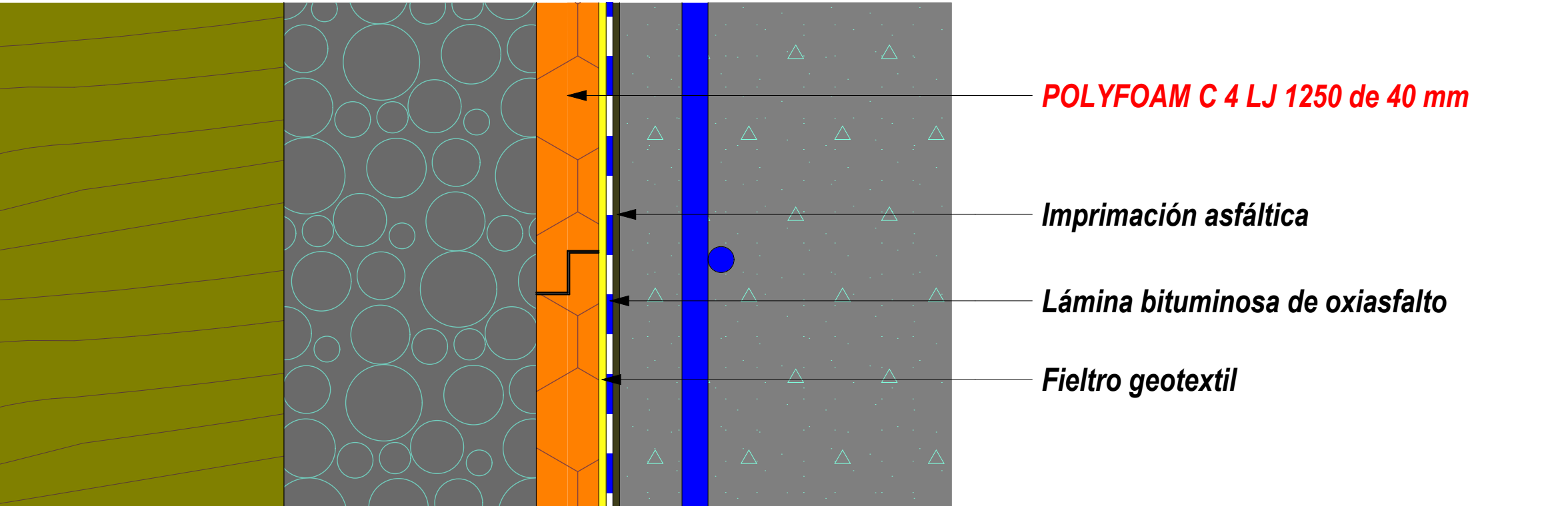
MURO ENTERRADO CON POLYFOAM C 4 LJ 1250
