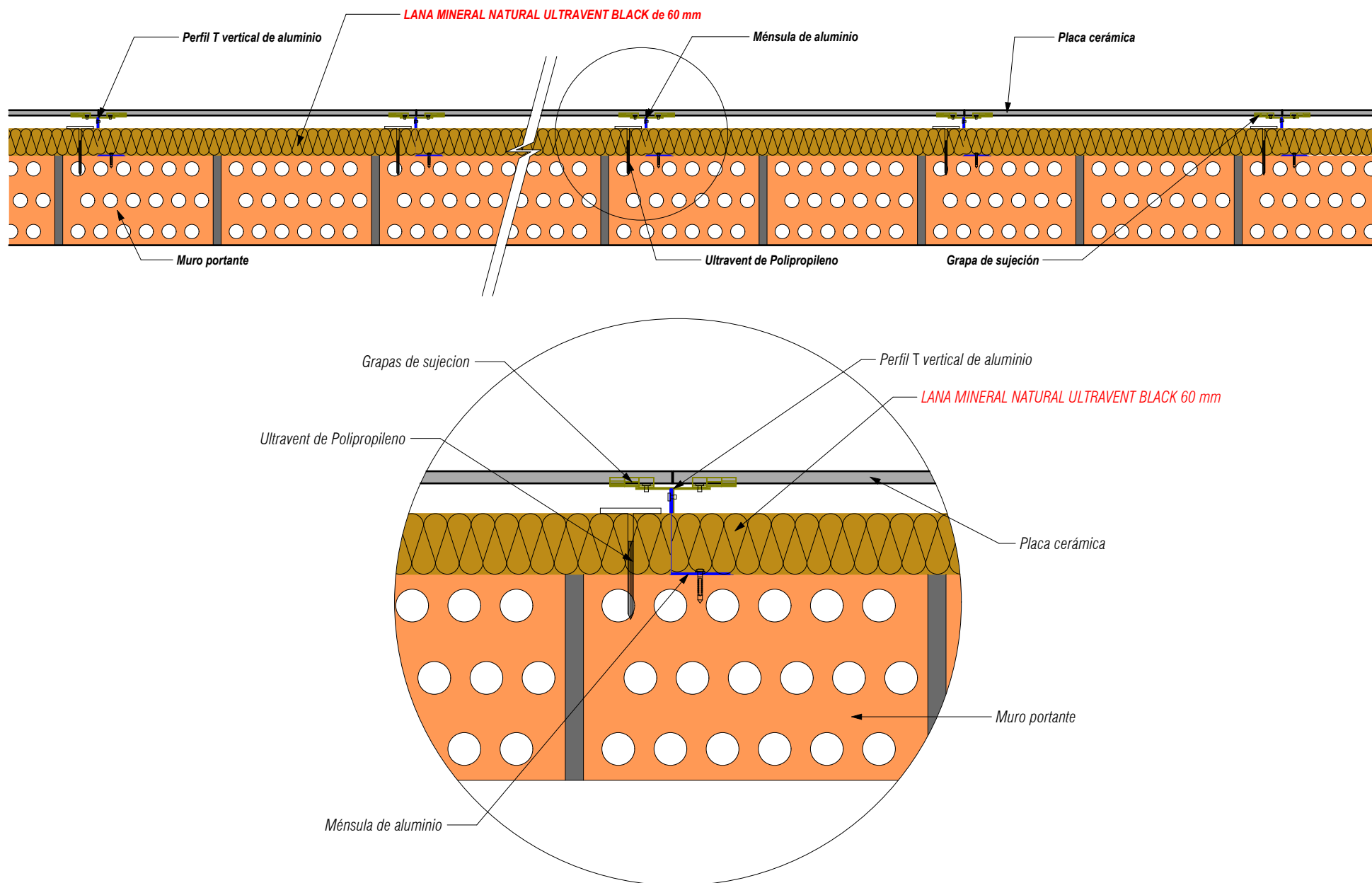
FACHADA VENTILADA CON ULTRAVENT BLACK
