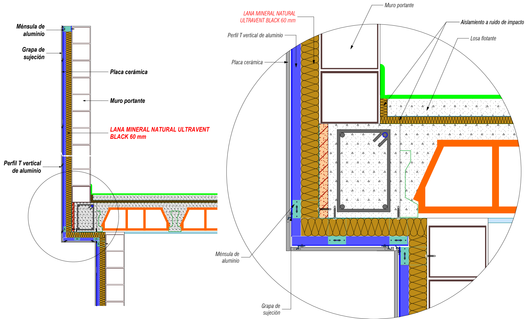
FACHADA VENTILADA CON ULTRAVENT BLACK
