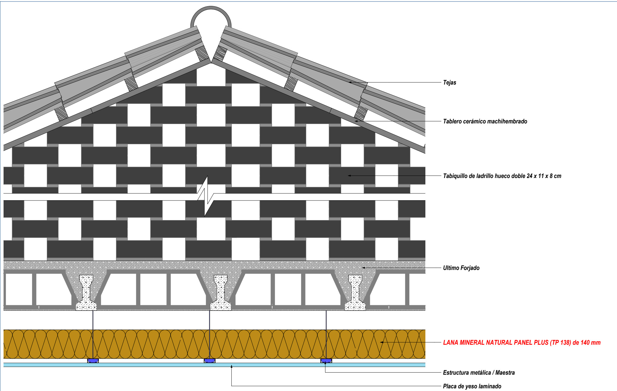
AISLAMIENTO INTERIOR BAJO ULTIMO FORJADO CON LANA MINERAL NATURAL PANEL PLUS (TP 138)
