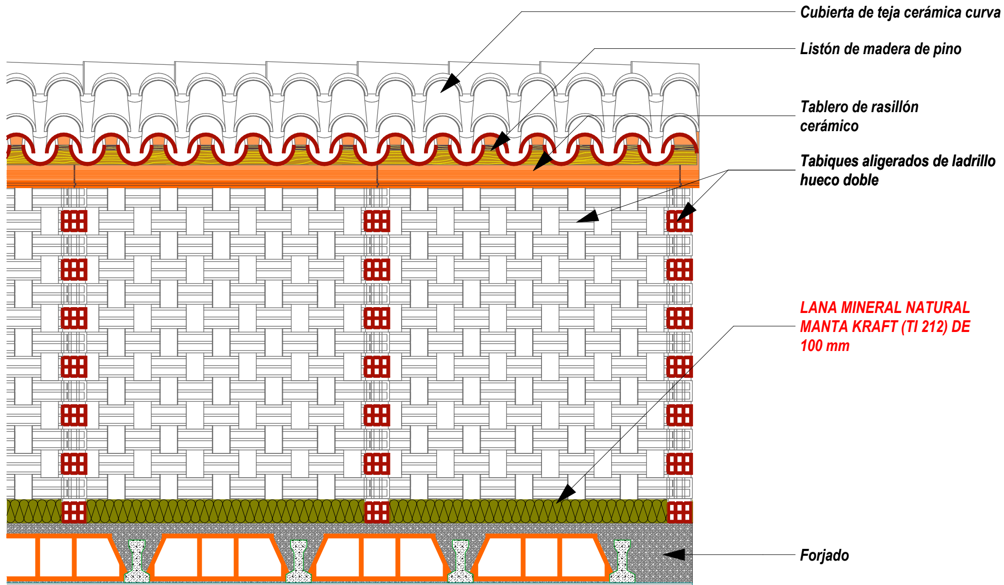
CUBIERTA INCLINADA SOBRE TABIQUILLOS CON MANTA KRAFT (TI 212)
