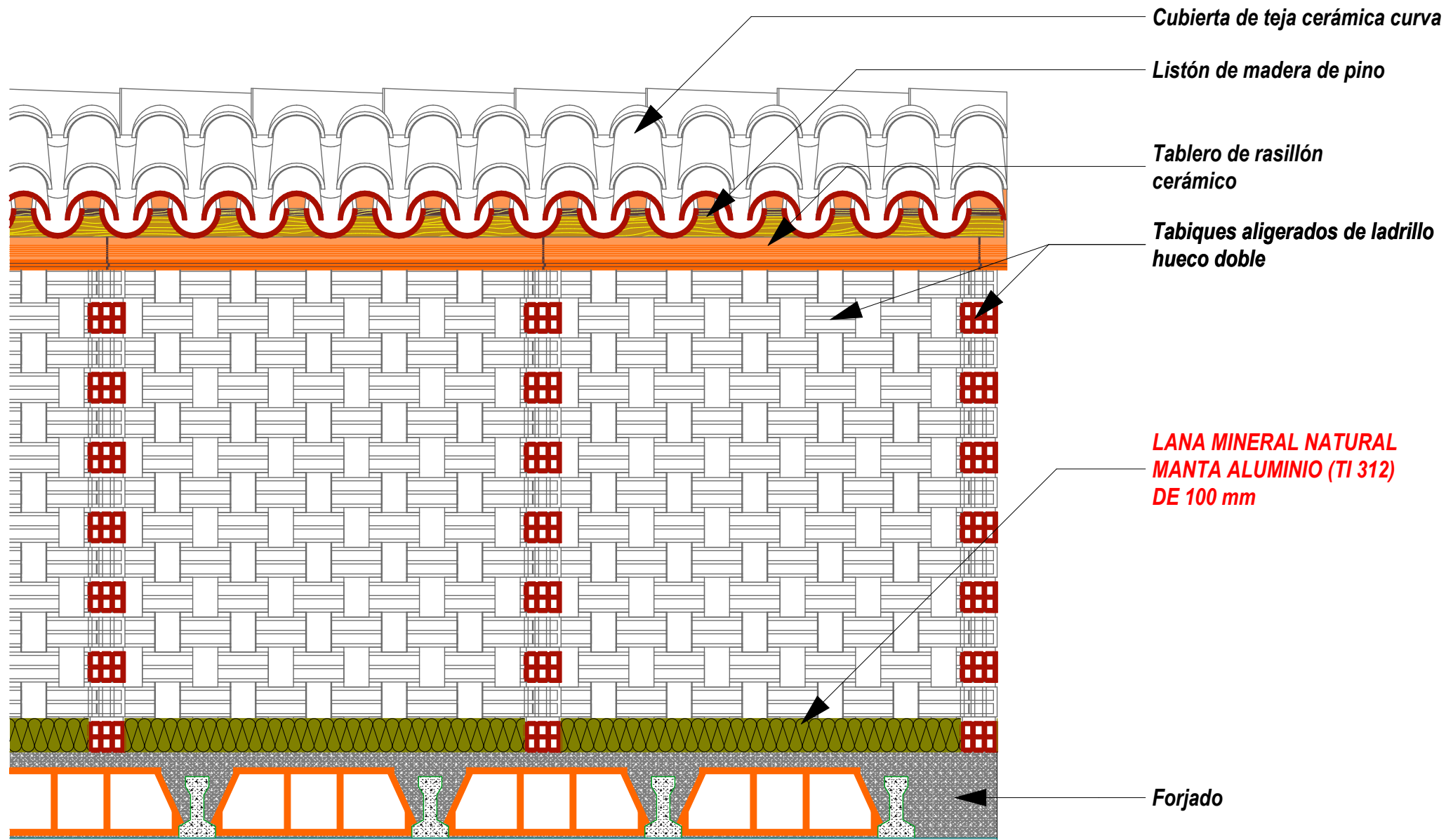
CUBIERTA INCLINADA SOBRE TABIQUILLOS CON MANTA ALUMINIO (TI 312)
