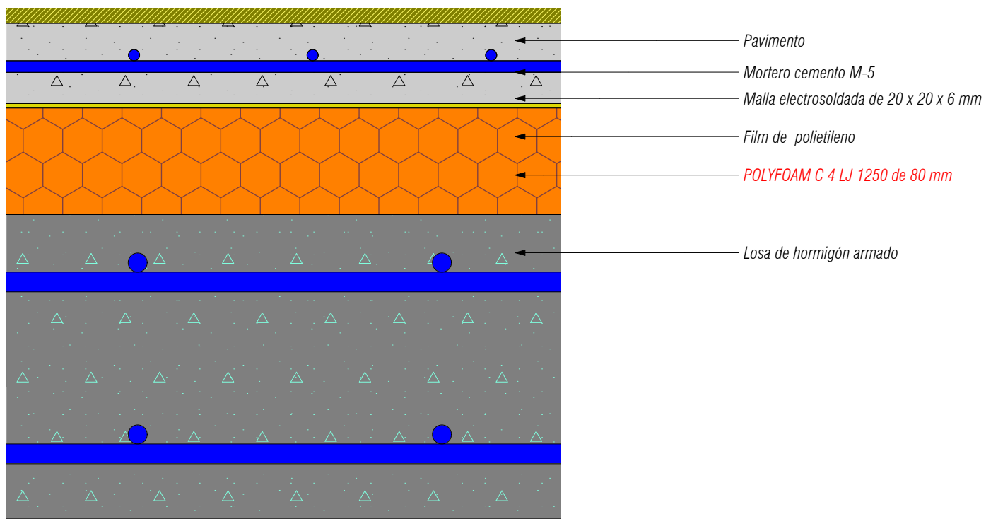
DETALLE 01
