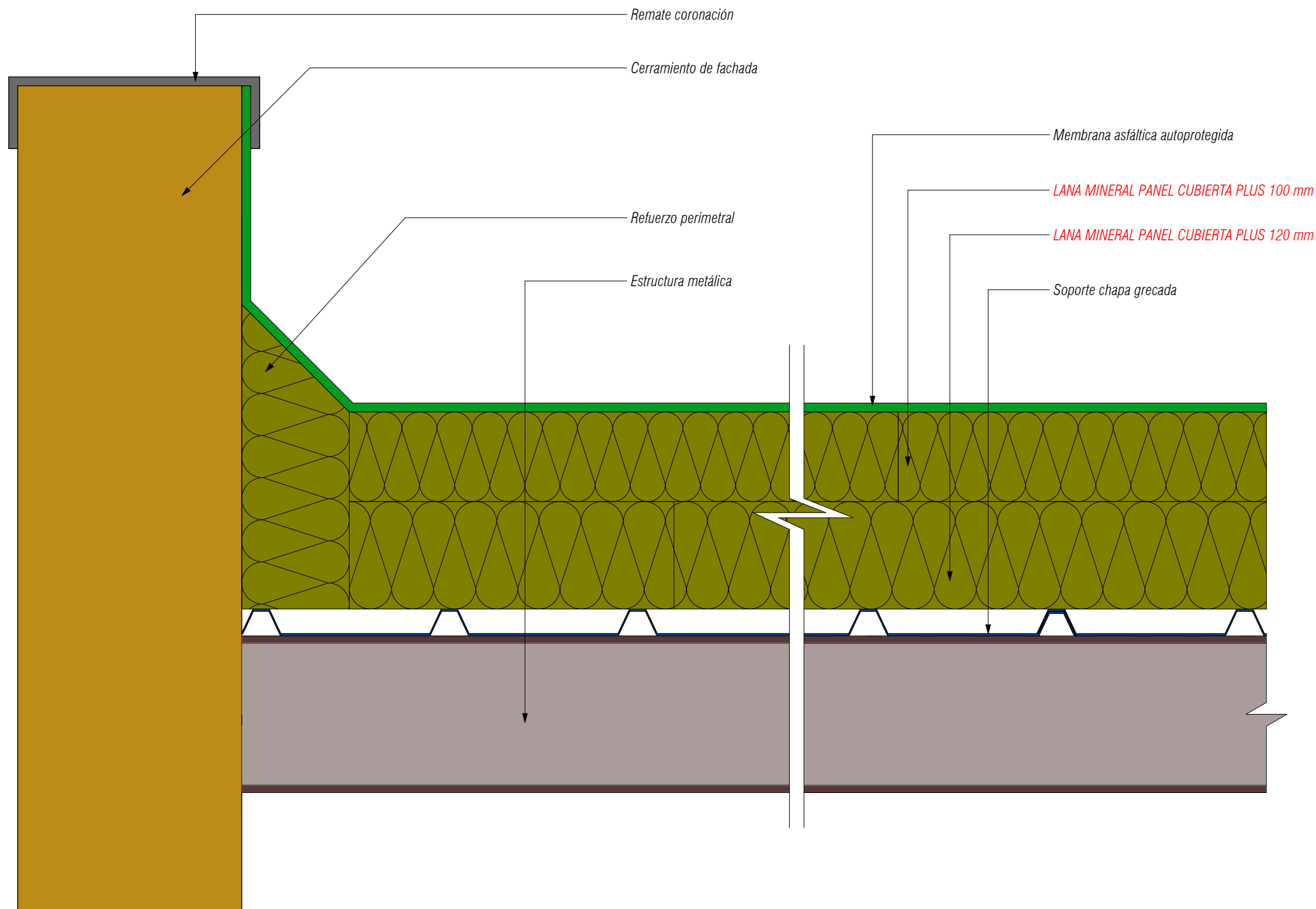
CUBIERTA DECK CON PANEL CUBIERTA PLUS
