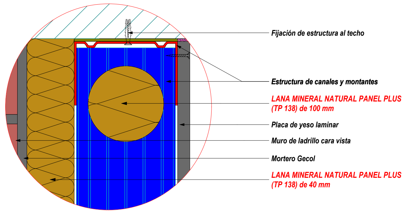
DETALLE - 3
