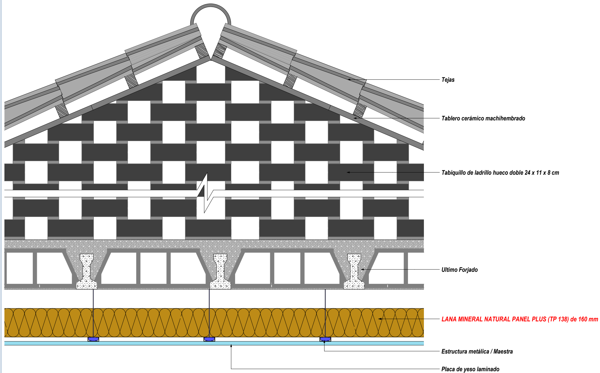
AISLAMIENTO INTERIOR BAJO ULTIMO FORJADO CON LANA MINERAL NATURAL PANEL PLUS (TP 138)
