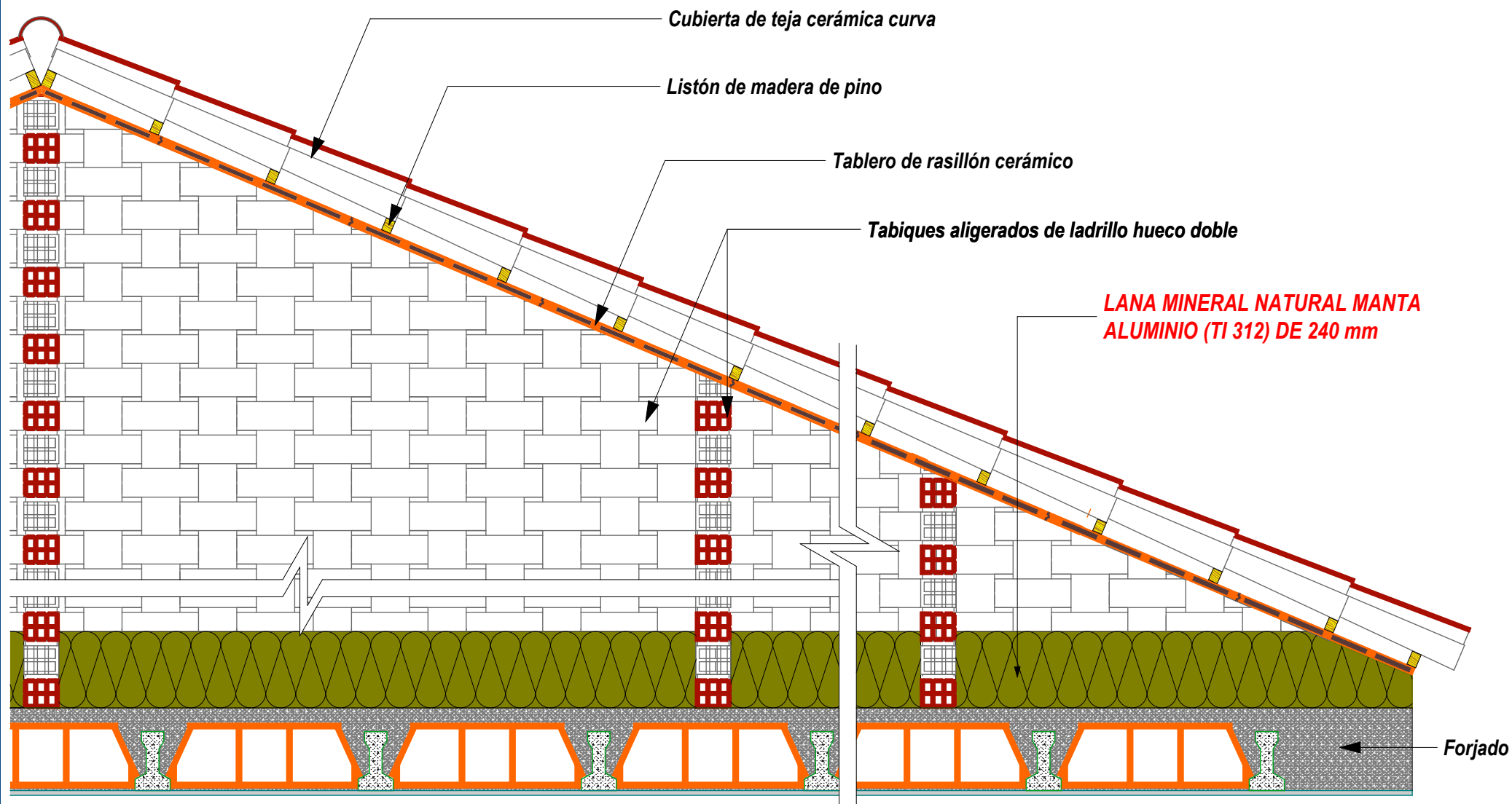
CUBIERTA INCLINADA SOBRE TABIQUILLOS CON MANTA ALUMINIO (TI 312)
