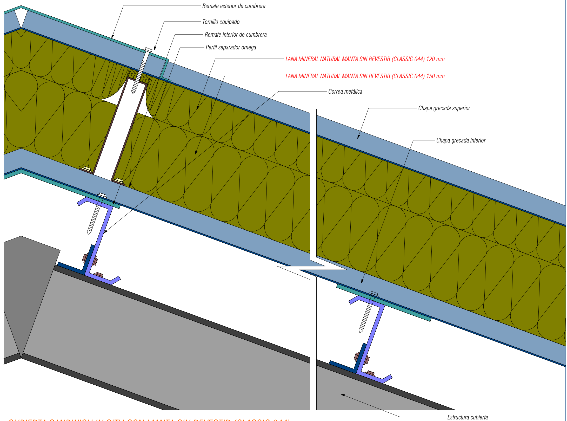
CUBIERTA SANDWICH IN SITU CON MANTA SIN REVESTIR (CLASSIC 044)
